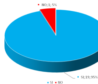
Figura 125. Conseguitamento obiettivi di qualità ambientale per lo stato chimico dei fiumi -Puglia.
