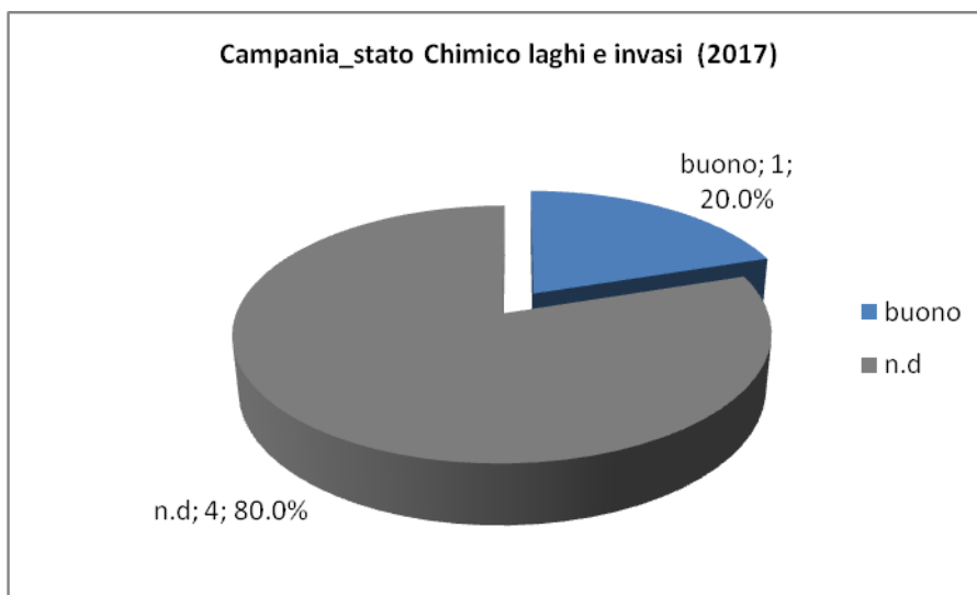
Figura 53. Stato chimico dei laghi della Campania.
