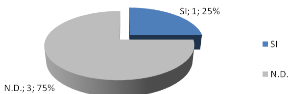
Figura 116. Conseguitamento obiettivi di qualità ambientale per lo stato ecologico dei laghi - Campania.
