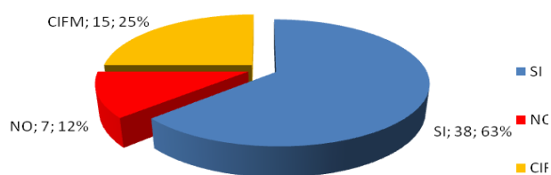
Figura 114. Conseguitamento obiettivi di qualità ambientale per lo stato ecologico delle acque marino-costiere - Campania.
