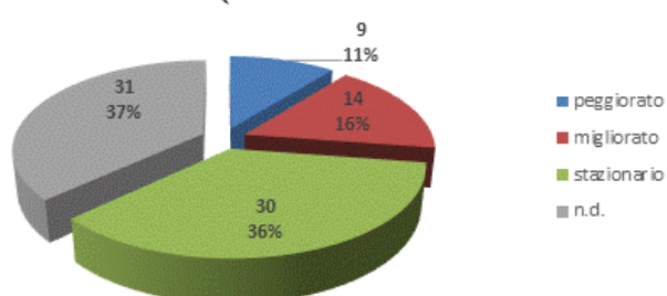
Figura 31. Trend stato ecologico fiumi della Basilicata. Trend stato ecologico C.I. fluviali aggiornato Basilicata
