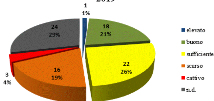
Figura 29. Stato ecologico dei fiumi della Basilicata.
