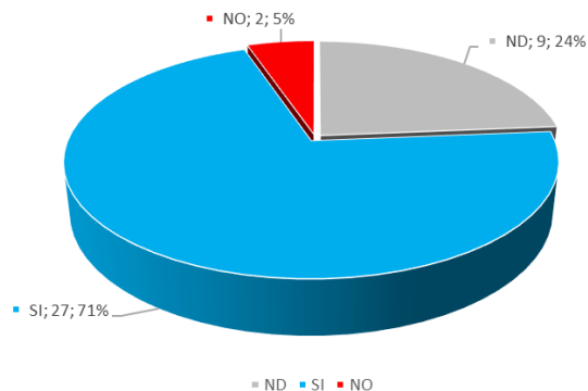
Figura 121. Conseguitamento obiettivi di qualità ambientale per lo stato chimico dei fiumi - Lazio.
