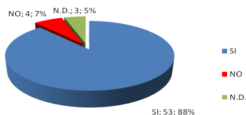
Figura 115. Conseguitamento obiettivi di qualità ambientale per lo stato chimico delle acque marino-costiere - Campania.
