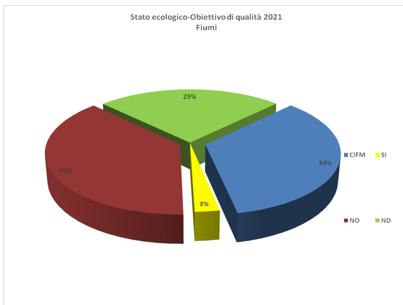
Figura 110. Conseguitamento obiettivi di qualità ambientale per lo stato ecologico dei fiumi - Calabria.
