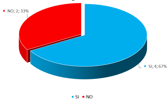
Figura 130. Conseguimento obiettivi di qualità ambientale per lo stato ecologico delle acque di transizione -Puglia.
